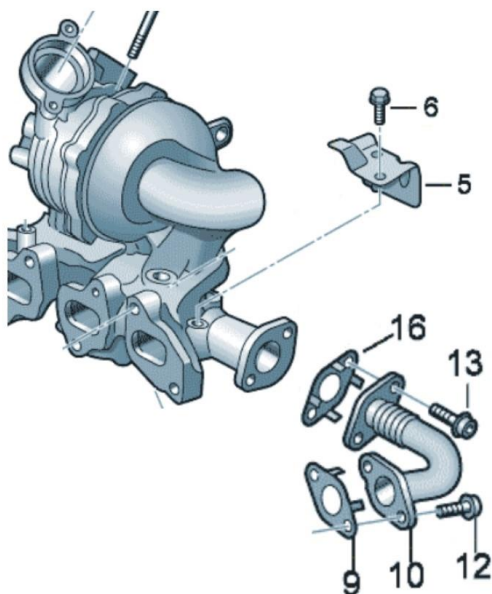
Rys. 2. Schemat elementów adaptacyjnych wymaganych przy montażu (pozycje: 5, 6, 9, 10, 12, 13, 16).
